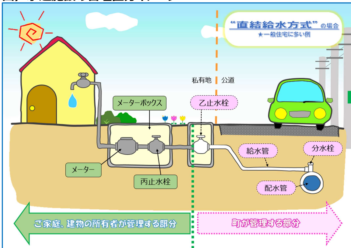
図) 水道施設の管理区分イメージ
