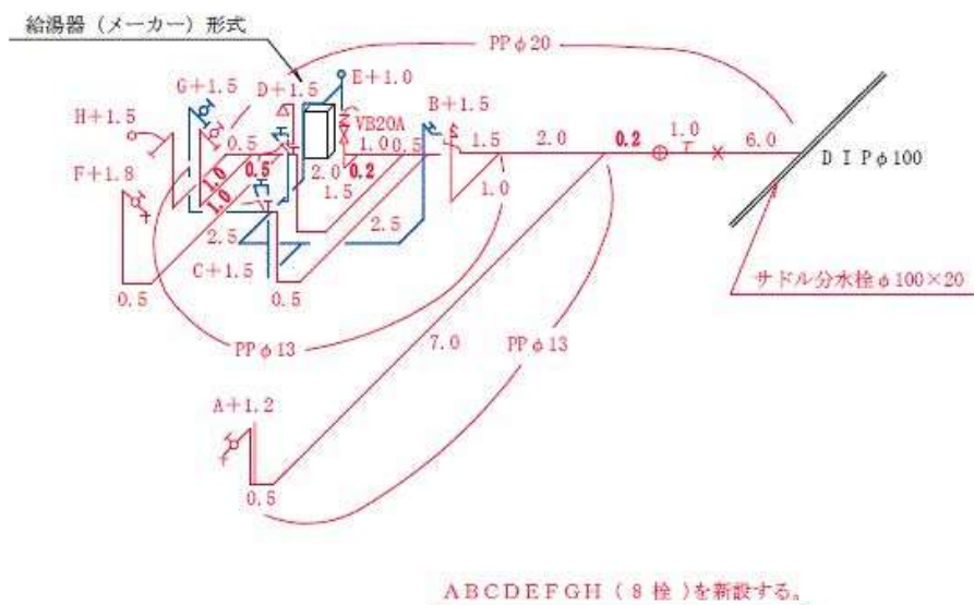
立面図
